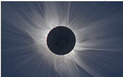
sluneční korona - paprsky vedle zakrytého slunce = sluneční korona, která je extrémně horká, teplota 2 mil. stupňů
